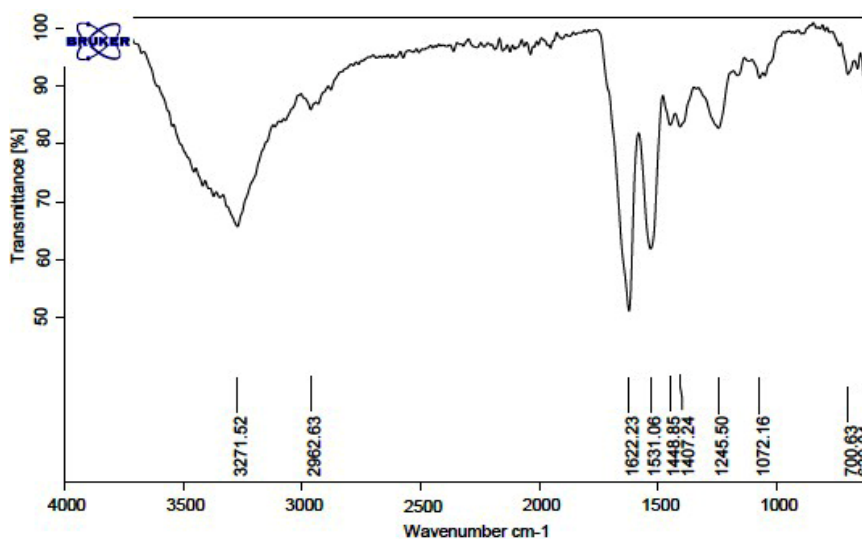
Fig. 2. FT-IR (ATR) spectra of nano-ovalbumin.
