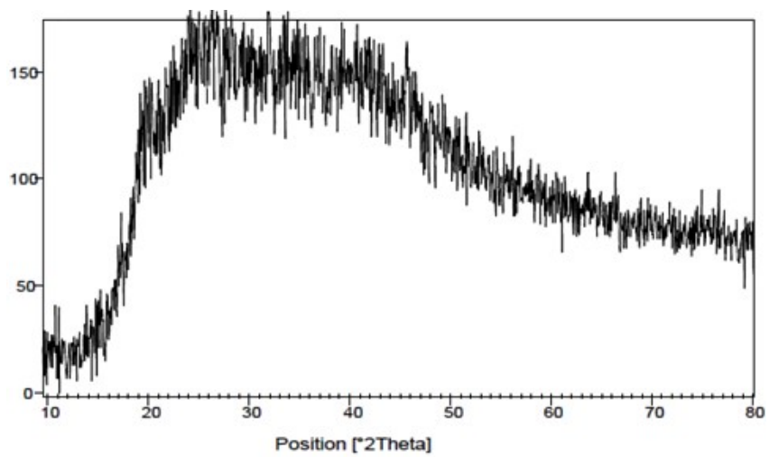
Fig. 6. XRD pattern of nano-ovalbumin.
